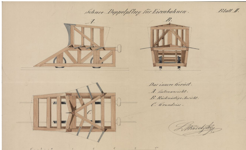
4. ábra: A hóeke szerkezeti rajzai Wodetzky szabadalmi leírásában
