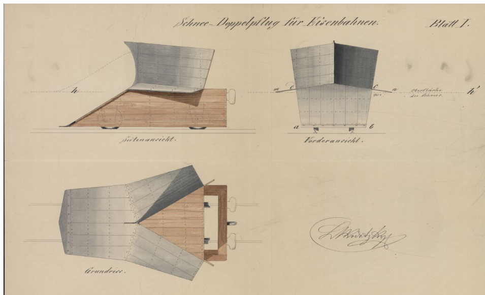
5. ábra: A hóeke fémborítása a szabadalmi leíráshoz mellékelt rajzon
